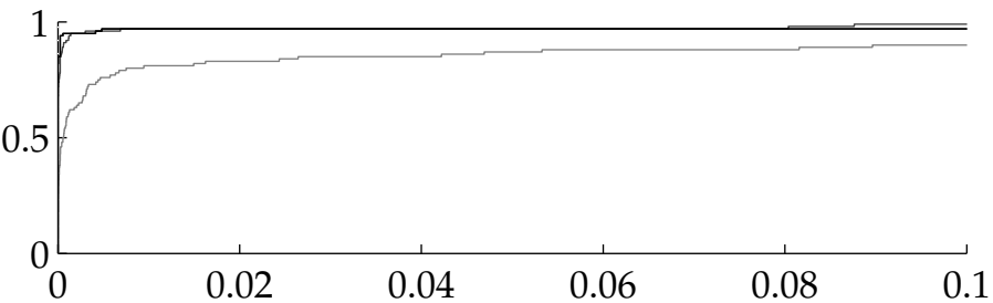
Nelder-Mead
